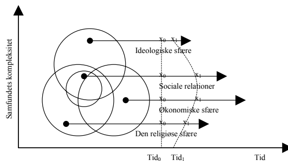
Figur 1: Vagn Wählins faseforskydningsmodel
